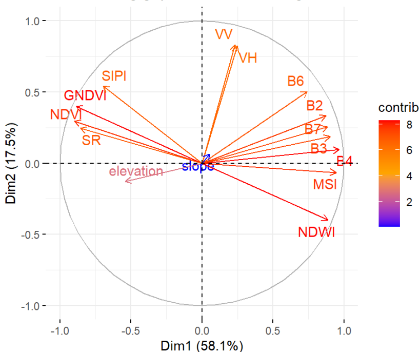
Hình 3.4. Biểu đồ biplot PCA
