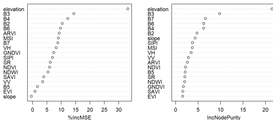
Hình 3.7. Mức độ quan trọng của các biến trong mô hình RF-All_var.
